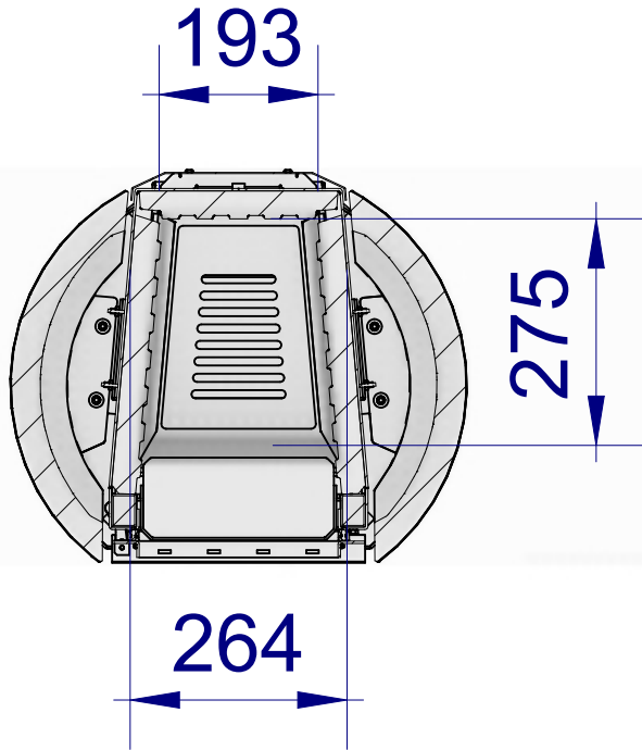
Feuerraum
